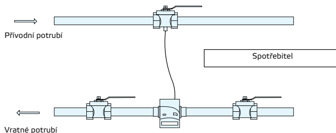
Symetrická instalace snímačů pro přístroj zelsius® C5-IUF se snímačem vratného toku vestavěným v měřicí kapsli
