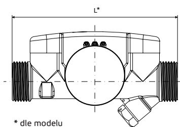
Symetrická instalace snímačů pro přístroj zelsius® C5-IUF se snímačem vratného toku vestavěným v měřicí kapsli
